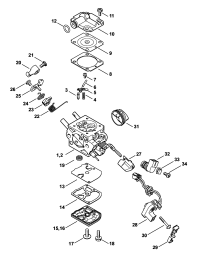
Karburátor
