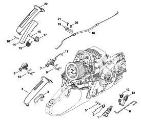
Ovládání plynu
