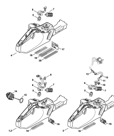
Těleso nádrže
