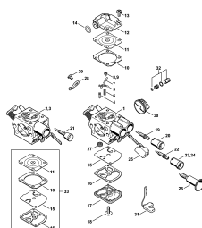
Karburátor C1Q-S254, C1Q-S213, C1Q-S180
