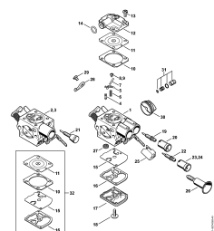
Karburátor C1Q-S253, C1Q-S212, C1Q-S179
