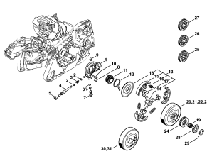
Olejové čerpadlo, spojka
