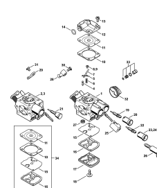
Karburátor C1Q-S211, C1Q-S178
