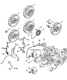
Zapalování, kabelový svazek
