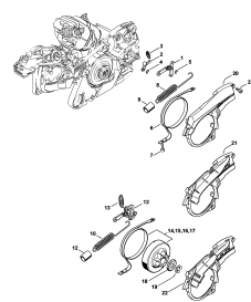
Řetězová brzda
