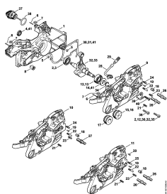
Kliková skříň
